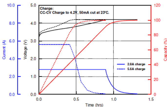
Charakterystyka ładowania akumulatora : MOLI INR18650-P28A 2800mAh
