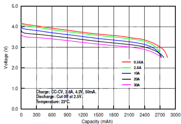
Charakterystyka rozładowania akumulatora : MOLI INR18650-P28A 2800mAh
